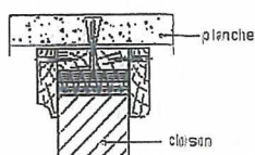
Liaison cloison-plancher (extrait des règles PS-MI)
